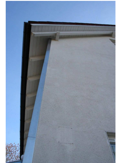
Blech-/Aluwinkel an Hausecken – verhindern das Festhalten der Spechte, wenn ausschließlich die Ecken behackt werden; Vorsicht: Die Dampfdiffusion des Wärmedämmverbundsystems darf nicht unterbunden werden!
